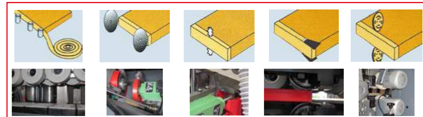
Kleben glueing
