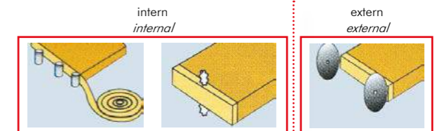
Kleben / glueing
